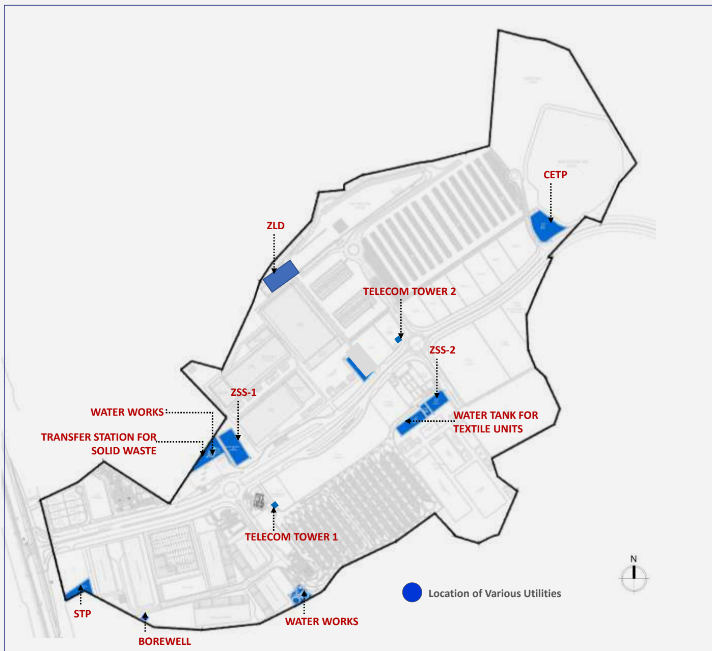
Figure 21 : Emplacement proposé des zones de services publics
